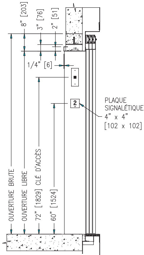
Élévation typique
