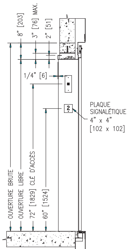
Élévation typique
