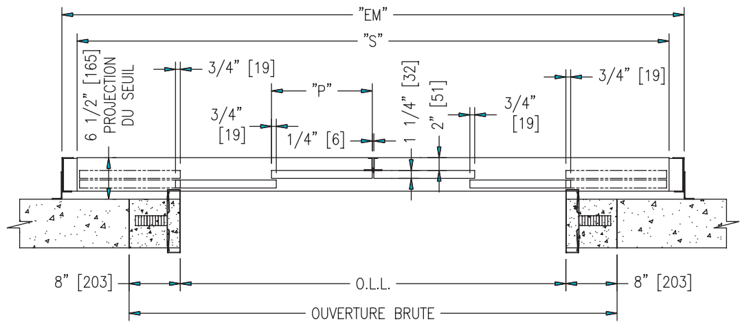
Vue en plan typique
