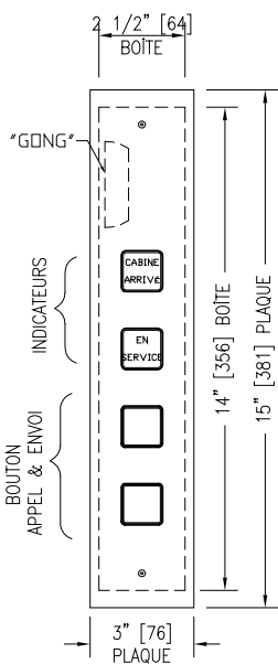
DÉTAIL BOÎTE À BOUTON
